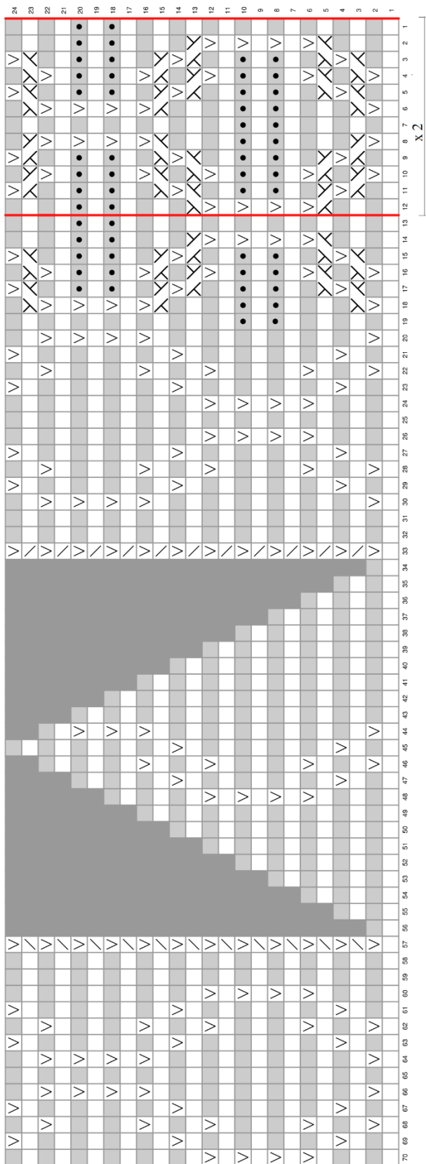
Схема Стопы А, размер S, правый носок
