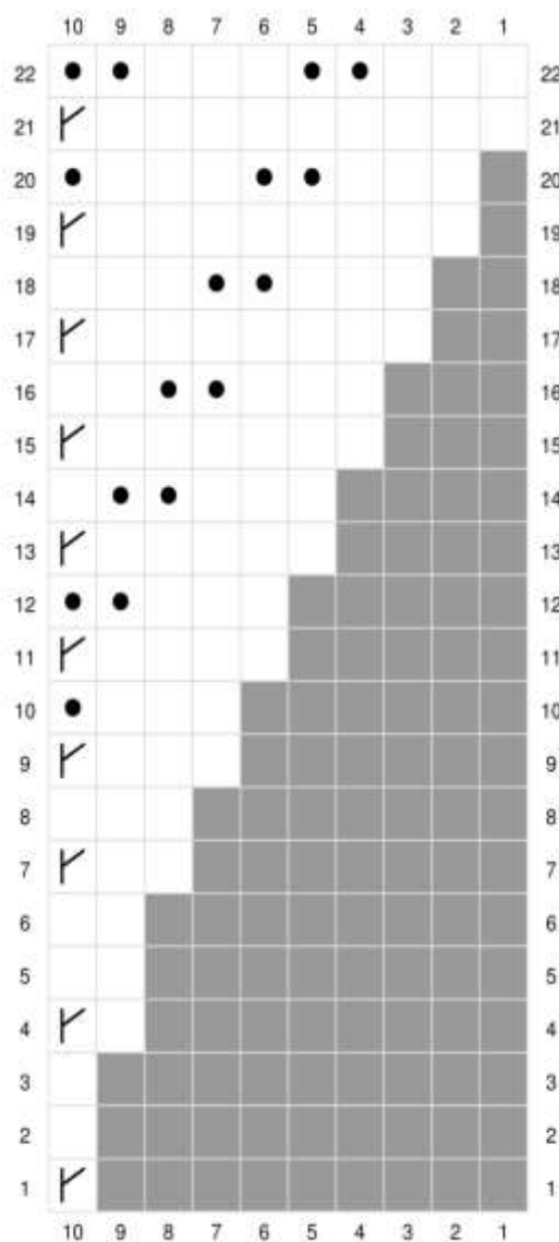
Схема 3-1 Узор Клина ЛП (СТw)
