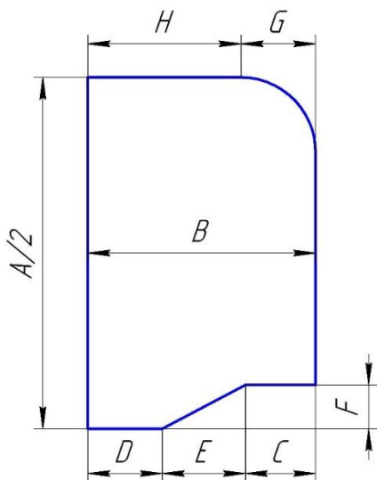
Схема капора
