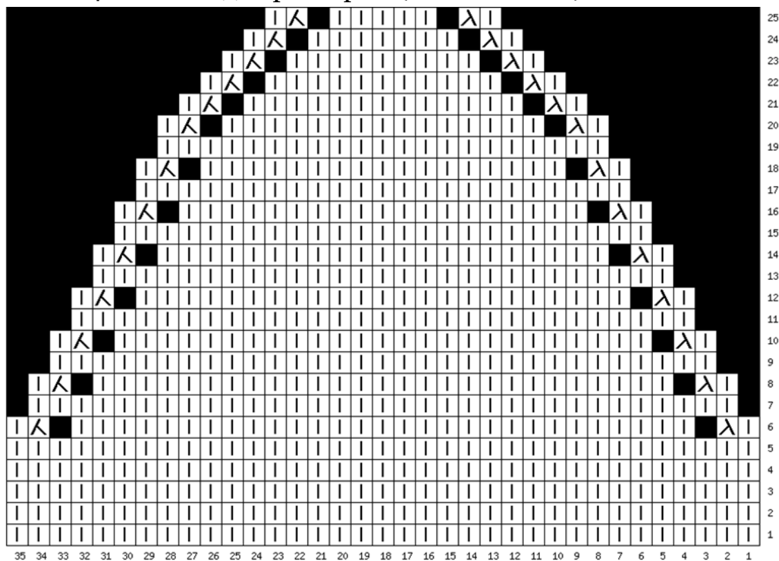
Схема 14.1. Мысок для размера 2 (нижняя часть)
