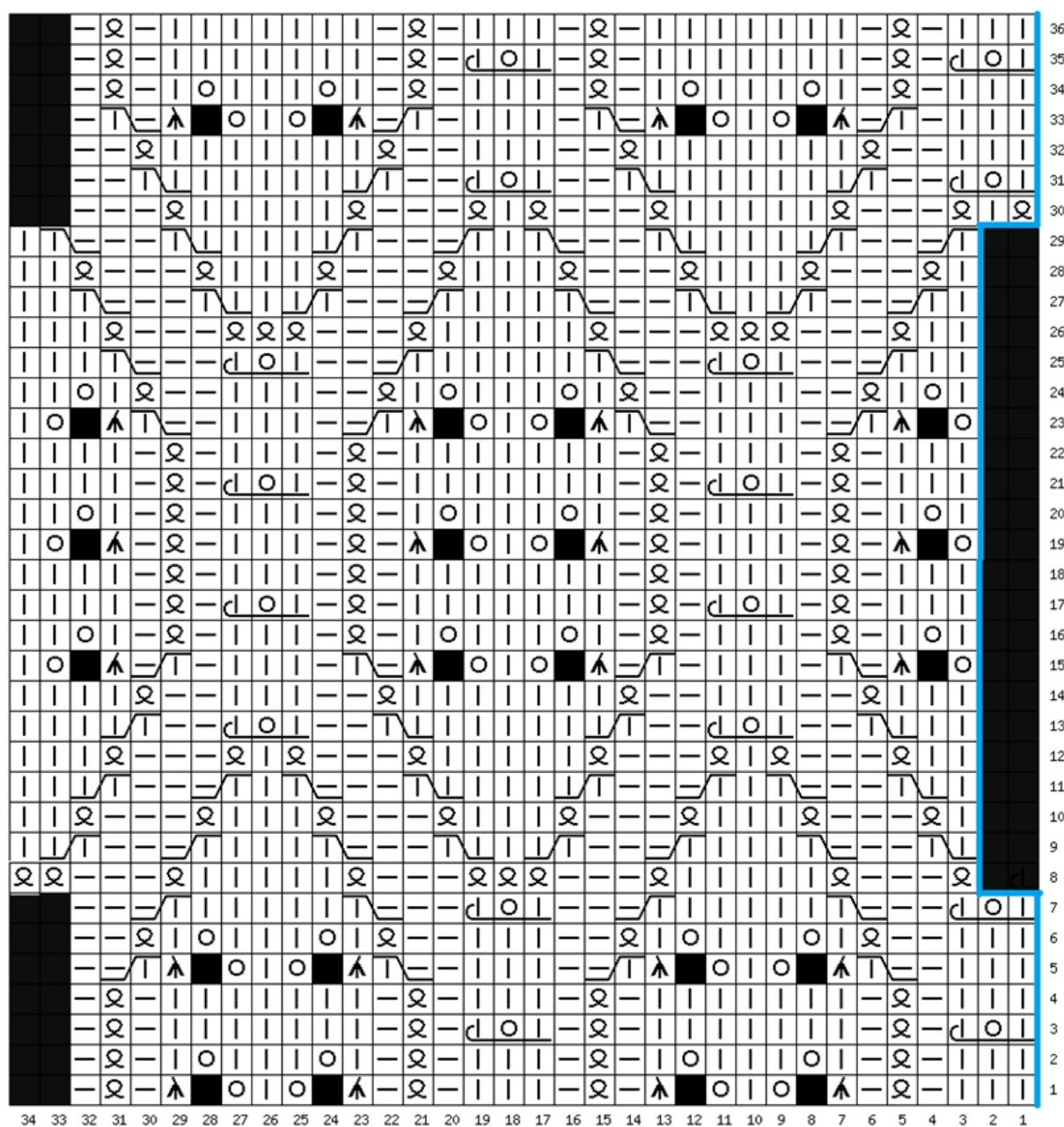
Схема 3. Паголенок для размера 1
