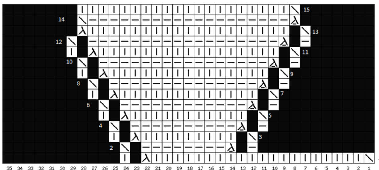
Схема 10. Пятка для размера 2
