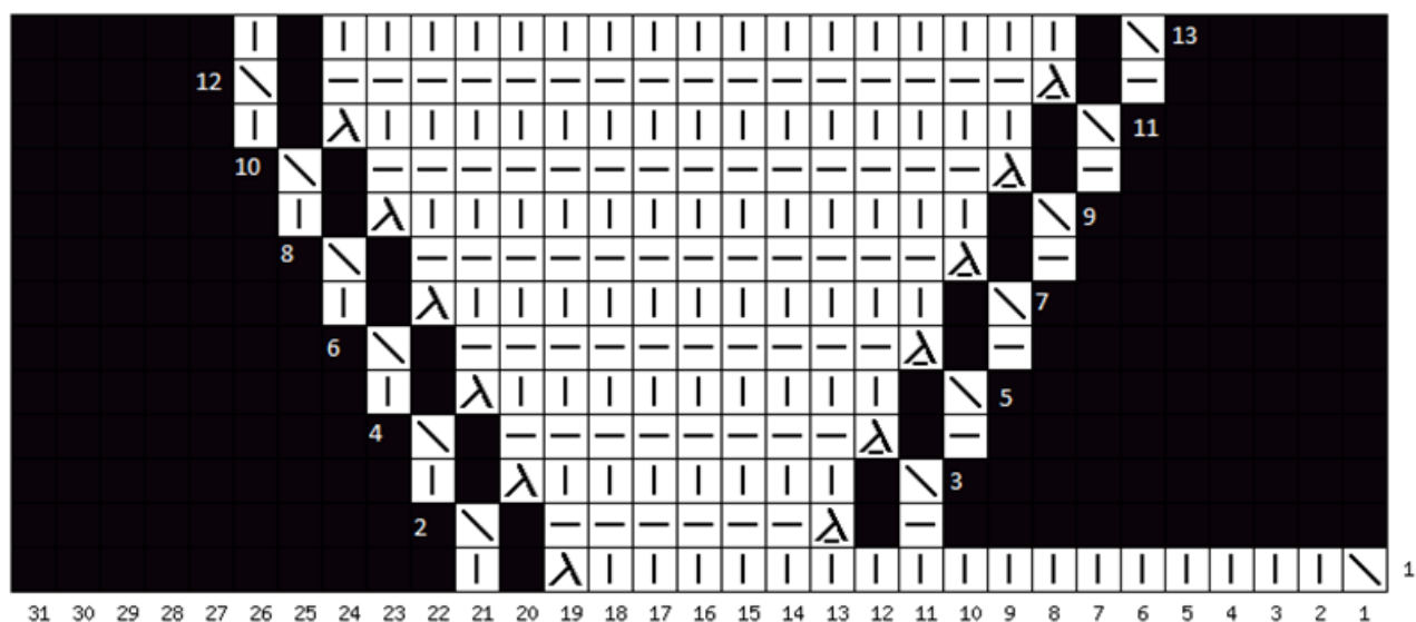
Схема 9. Пятка для размера 1
