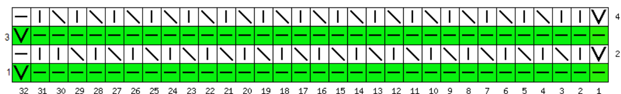
Схема 4.4 Стенка пятки для размера 2
