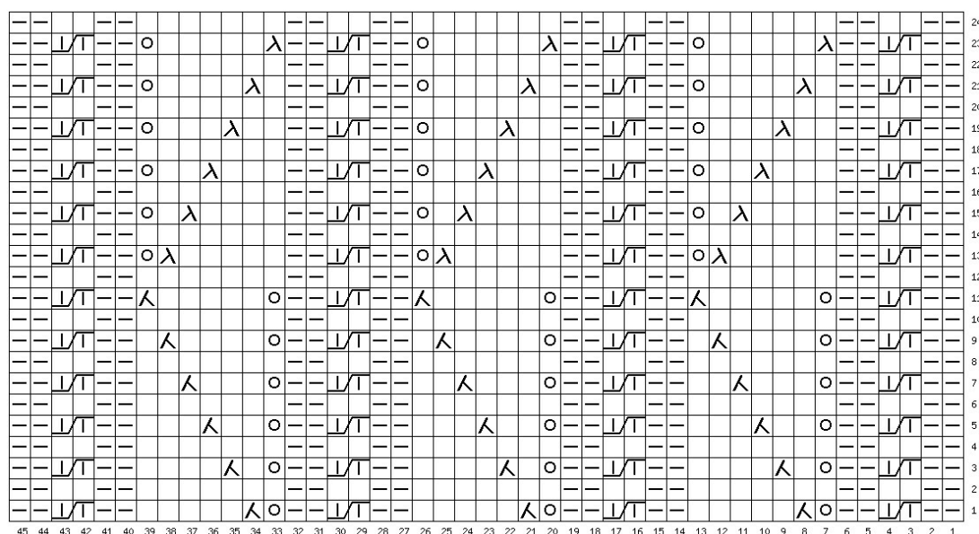
Схема 4.3
