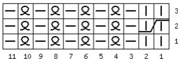
Схема 1.1
