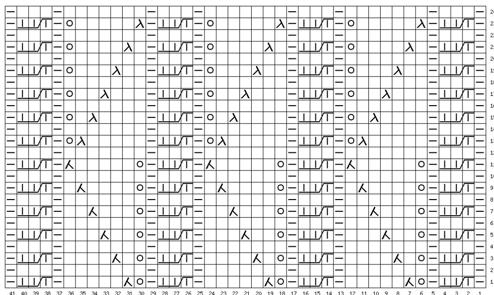
Схема 4.2
