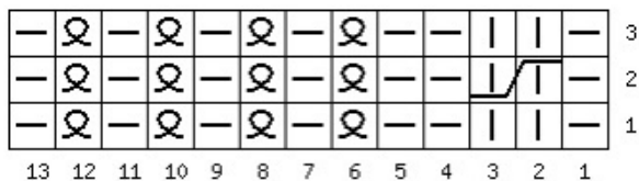
Схема 1.3
