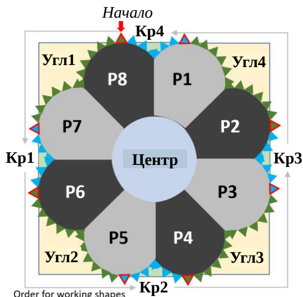
Рис. 8: Конструкция Фона блока
