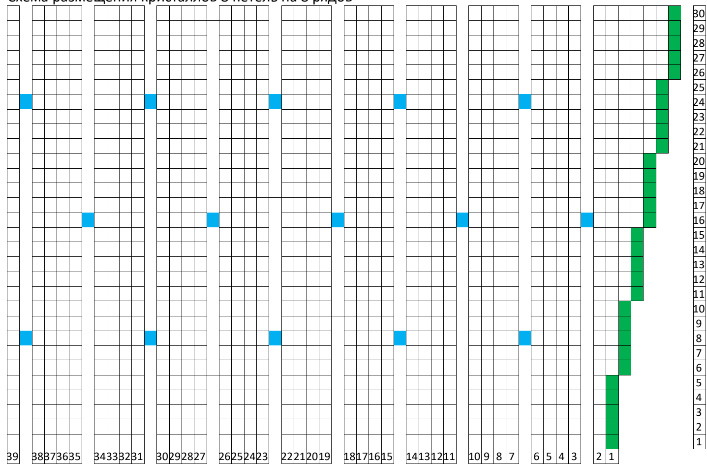
Схема размещения кристаллов 8 петель на 8 рядов
