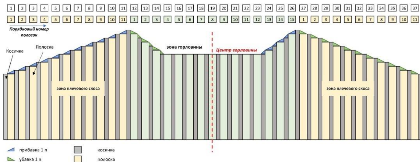
Рисунок 2. Схема детали «Спинка» для размера Medium при плотности – 19 п x 14 р в 10 см.
