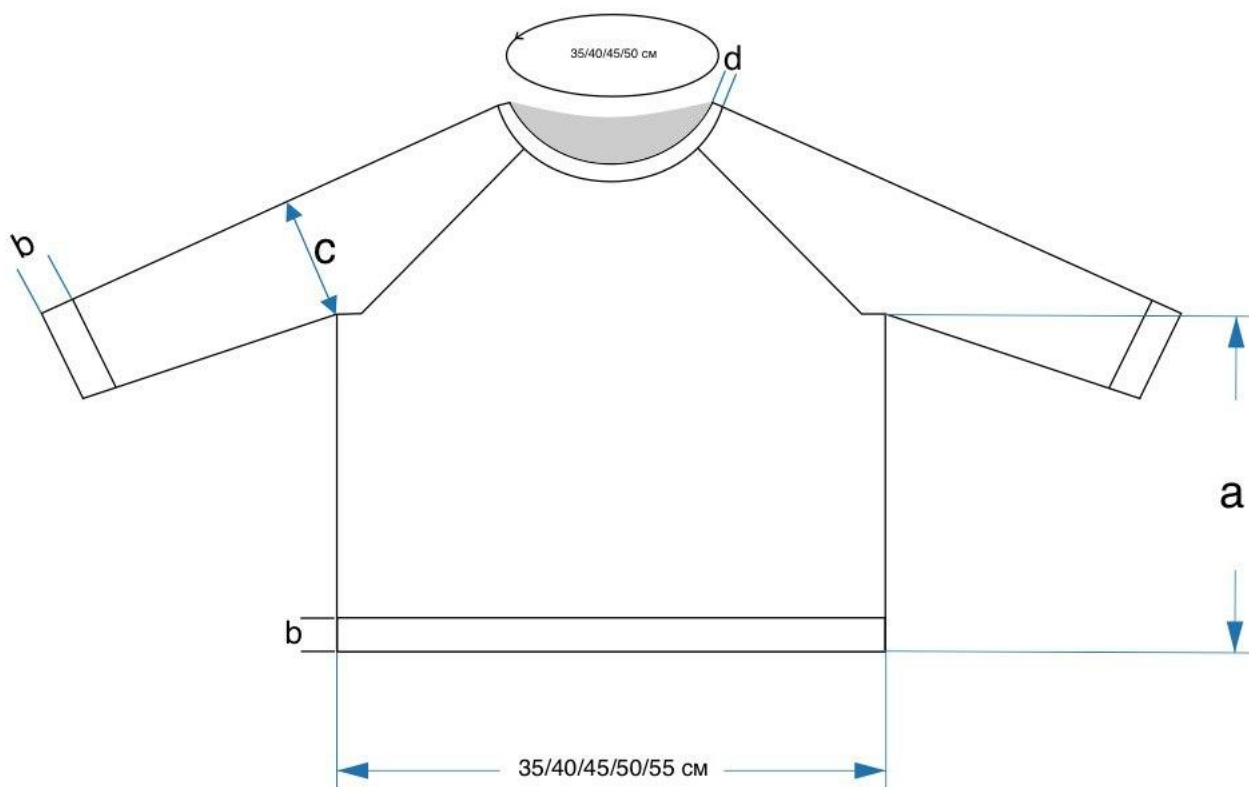
Рисунок 1 – Схема изделия
