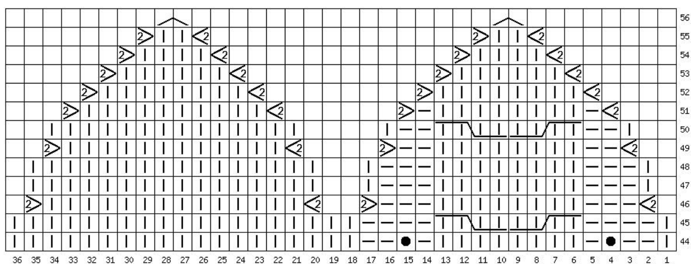
Схема макушки варежки
