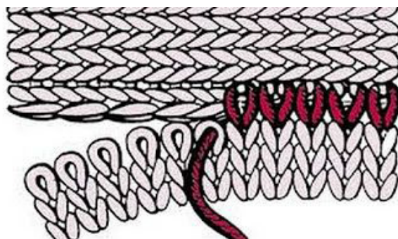
Прием вшивания рукава
