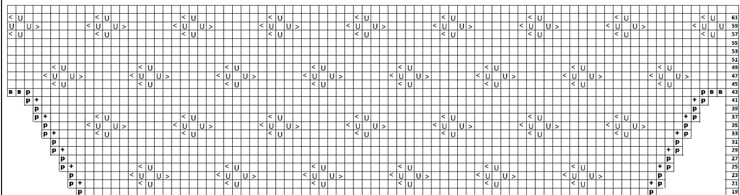
Схема спинки для размера XS
