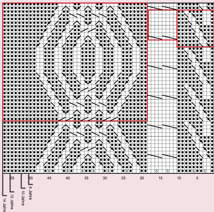
Strickschrift C (rechtes Vorderteil)
