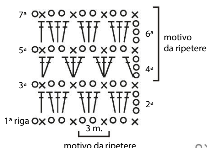
SCHEMA 1 -PUNTO FANTASIA
