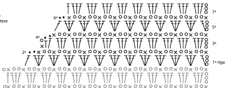
SCHEMA 2 -SCOLLO DAVANTI SINISTRO
