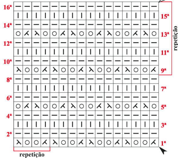
Diagrama 2 - Ponto fantasia (A)
