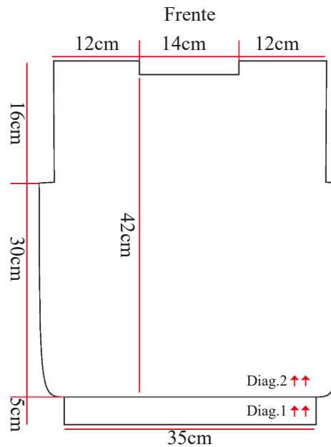
Esquema de medidas:
