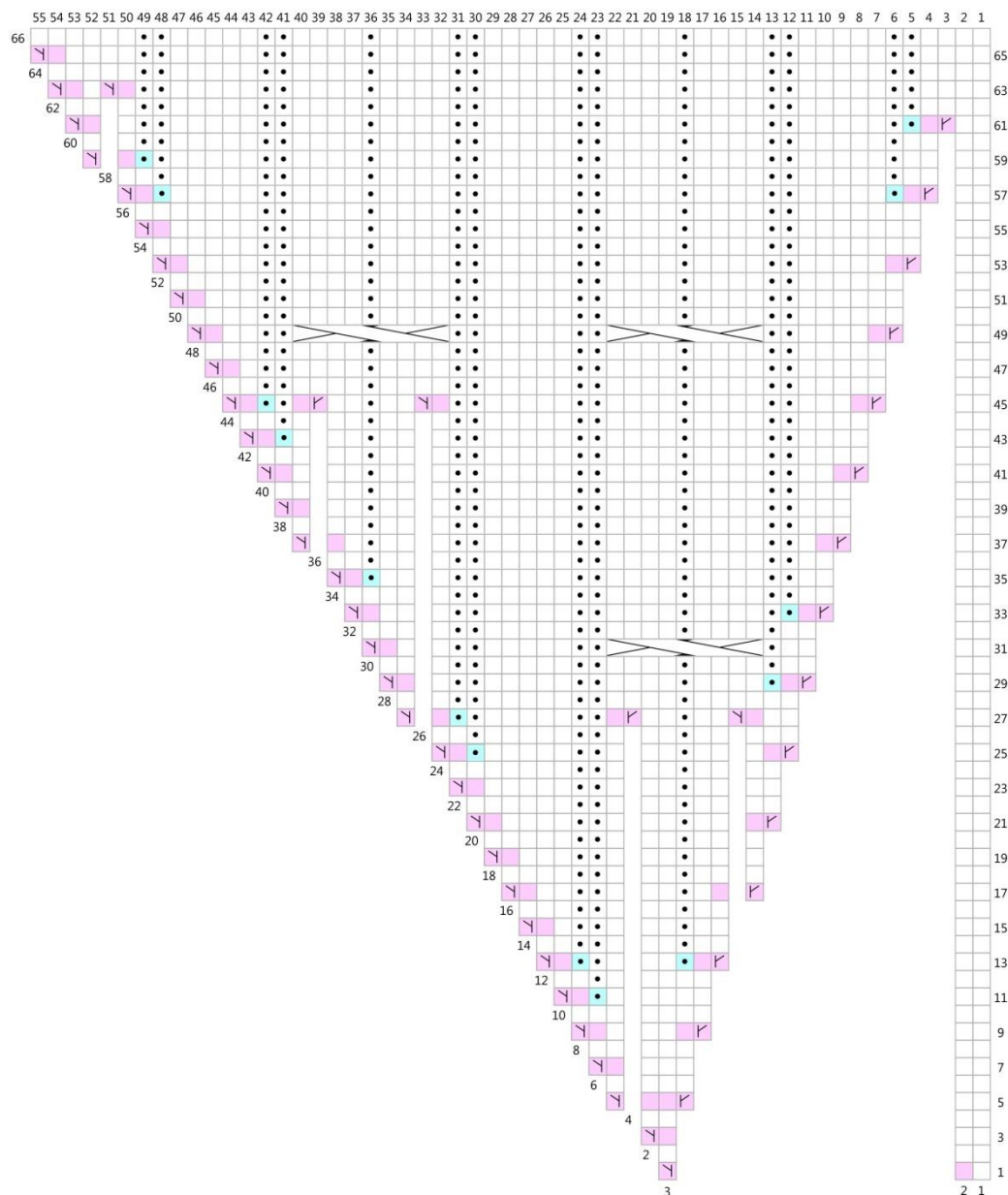
СХЕМА 2.1, РОЗМІР 4 (ЛІВА ЧАСТИНА ПЕРЕДУ)
