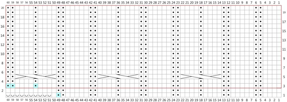
СХЕМА 3.2, РОЗМІР 2 (СПИНКА)
