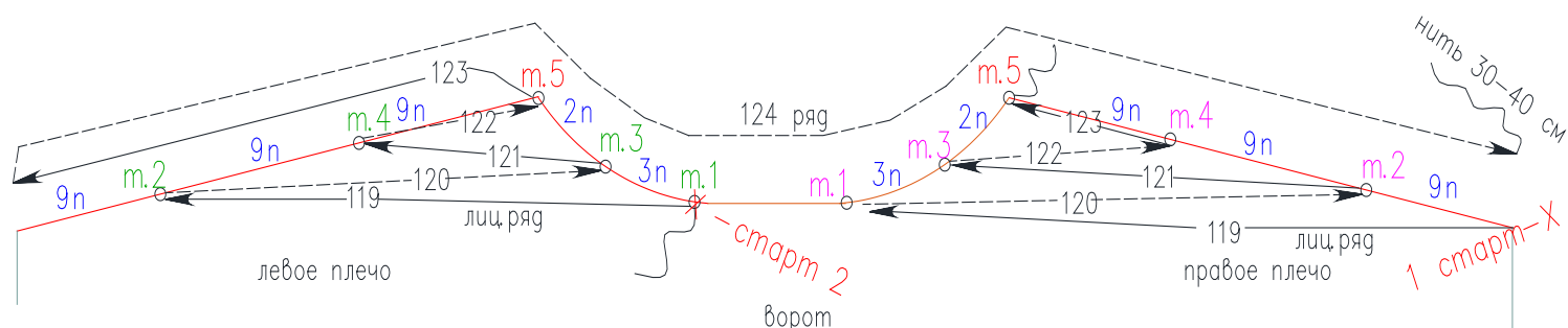
Схема 7: Скосы плечей и ворота спинки
