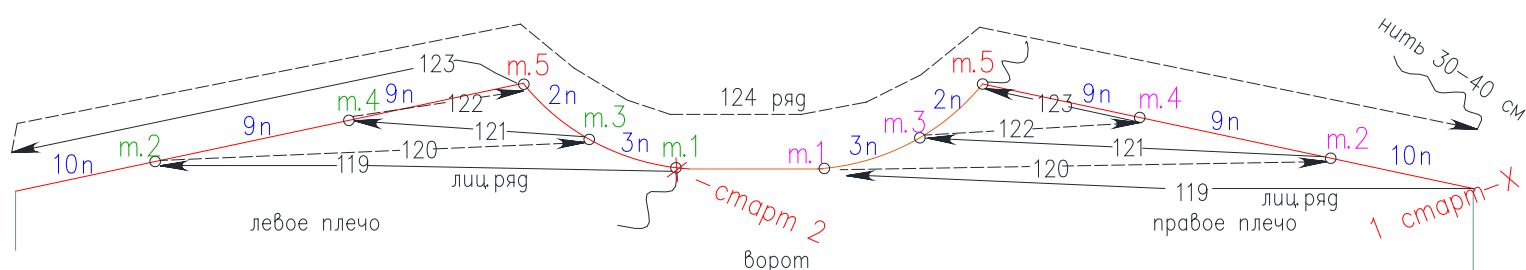
Схема 7: Скосы плечей и ворота спинки
