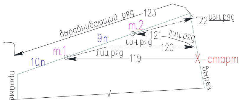
Схема 6: Скос правого плеча
