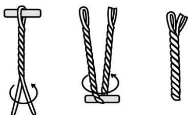
SCHEMA A - Cordoncino
