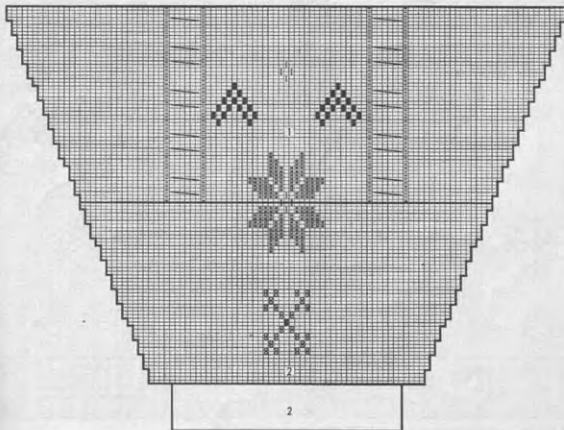
Схема (левый рукав)
