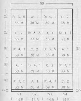
Чертеж-схема (перед) к модели 29
