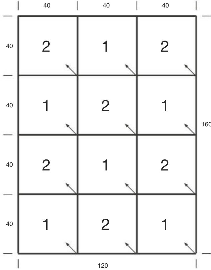
Схема соединения деталей к мод. 47
