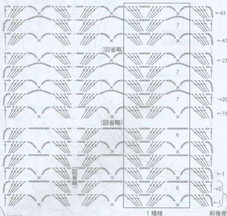
前身頃の模様編み B
