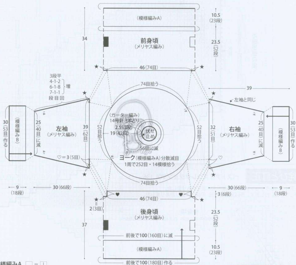
図省略 4目2段1模様 (作り目)
