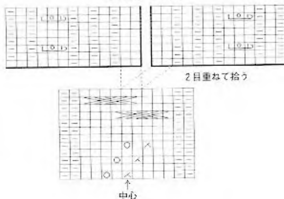
衿の拾い方
