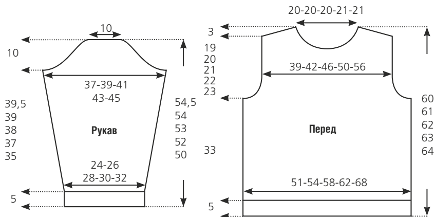
Счетная схема
