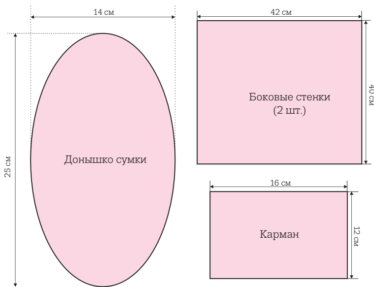
Рис. 21. Выкройка подкладки сумки
