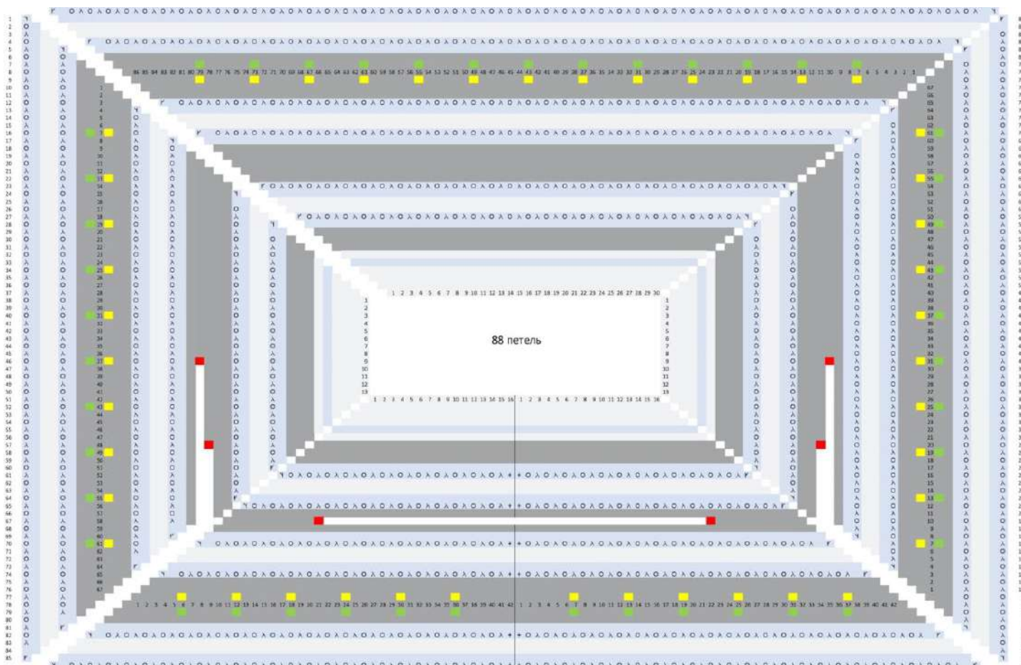
Схема реглана до отделения рукавов
