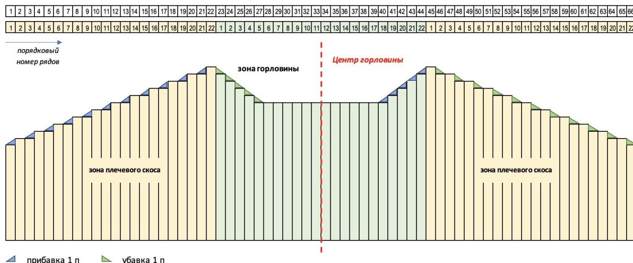
Рисунок 1. Схема детали «Спинка» для размера Medium при плотности – 17 п x 11 р в 10 см.
