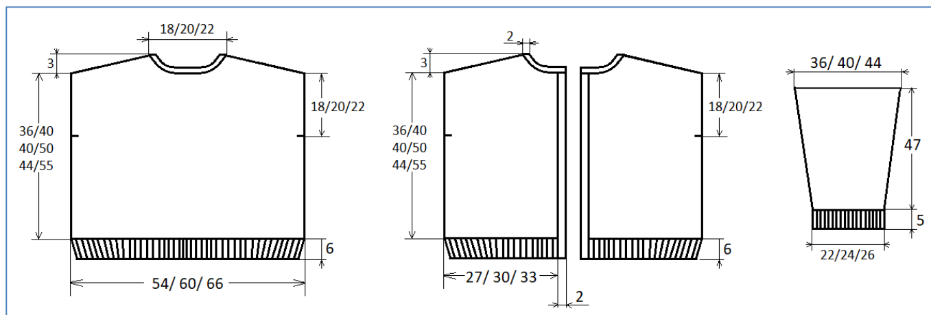
Чертеж 1.
