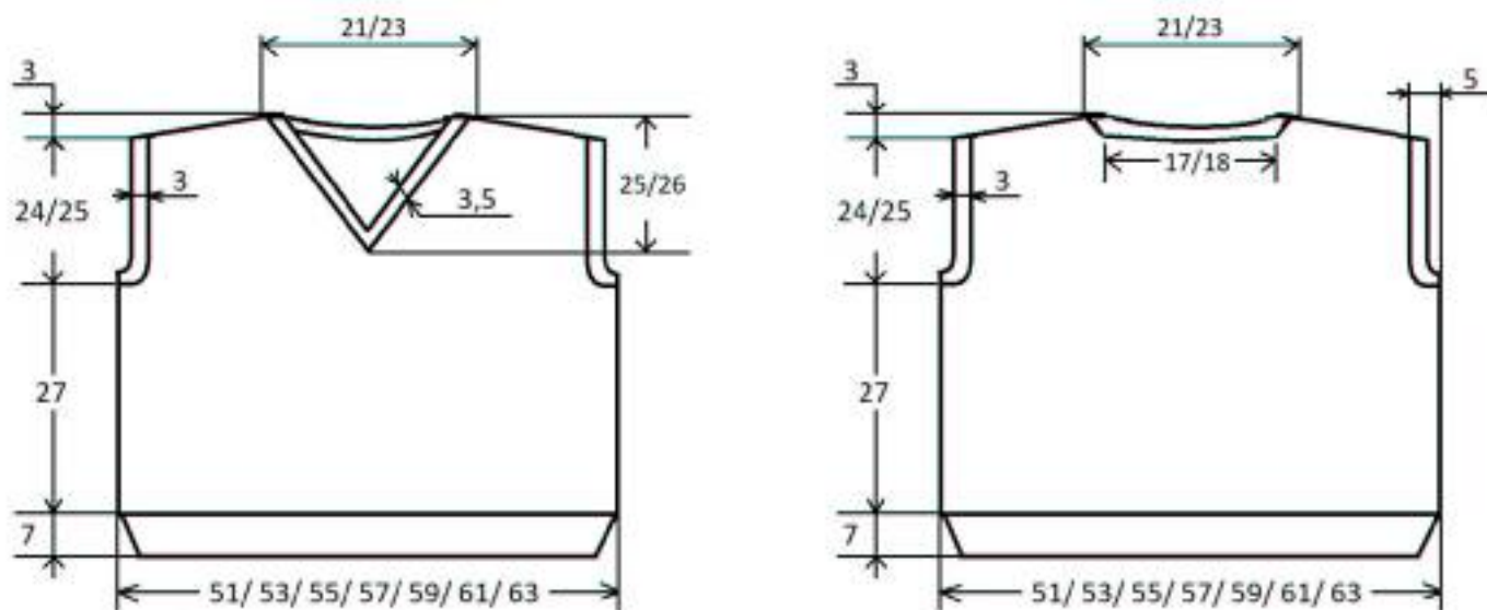
Чертеж 1.
