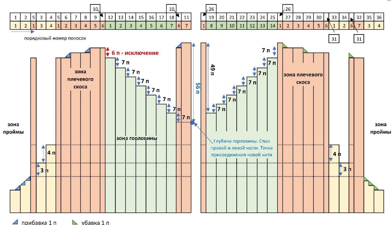
Рисунок 5. Измененная схема детали «Перед» для размера М при плотности – 20 п x 13 р в 10 см.
