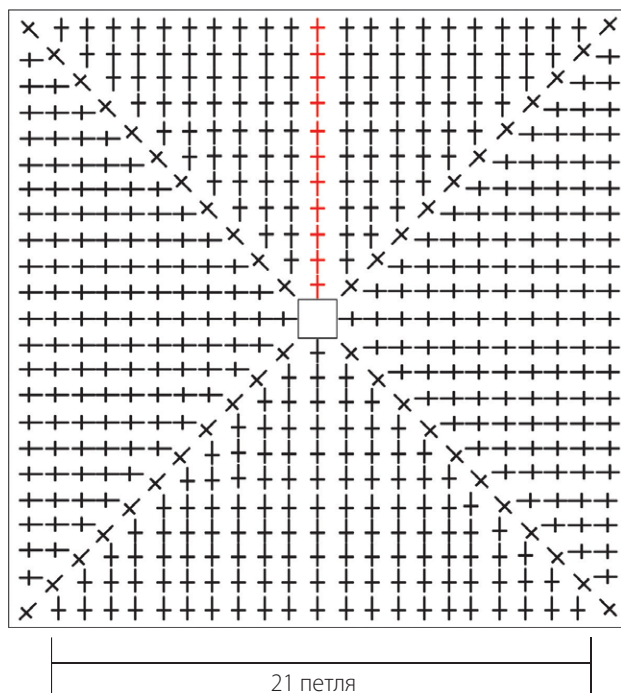
Схема квадрата
