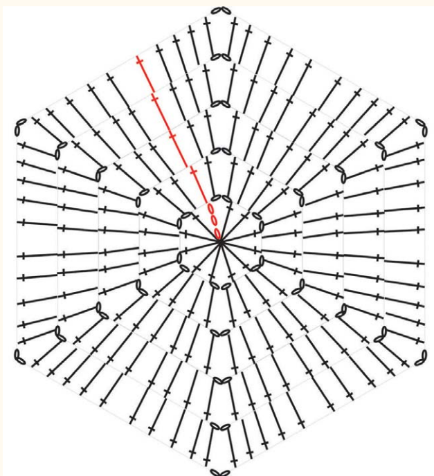
Схема элемента
